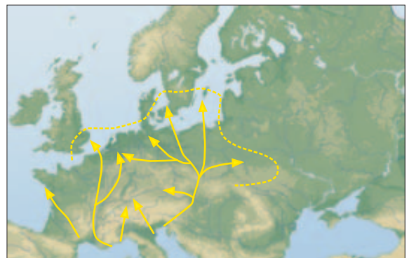
Abb. 5: Wahrscheinliche Einflugwege der Mittelmeermöwe nach Mitteleuropa im Sommer, basierend auf Ringfunden. Die gestrichelte Linie stellt die Nordgrenze des häufigen Vorkommens dar (aus KLEIN 2001). – Possible flyways of Yellow-legged Gulls into Central Europe in summer, based on ring recoveries. The broken line indicates the northern border of common and regular field observations (from KLEIN 2001).
